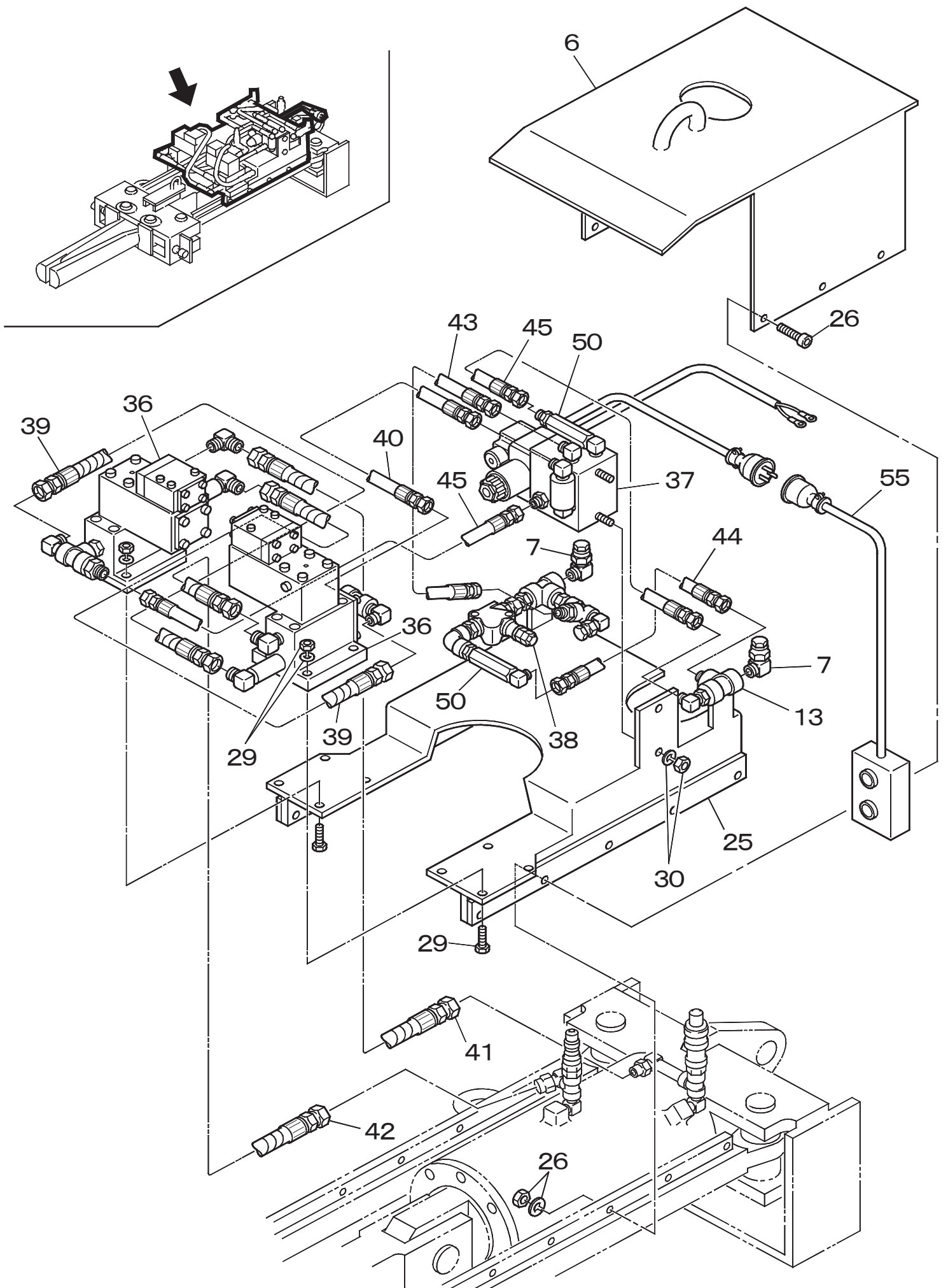
油圧割開機～リキヤ～『HUシリーズ』分解図(3/3)
