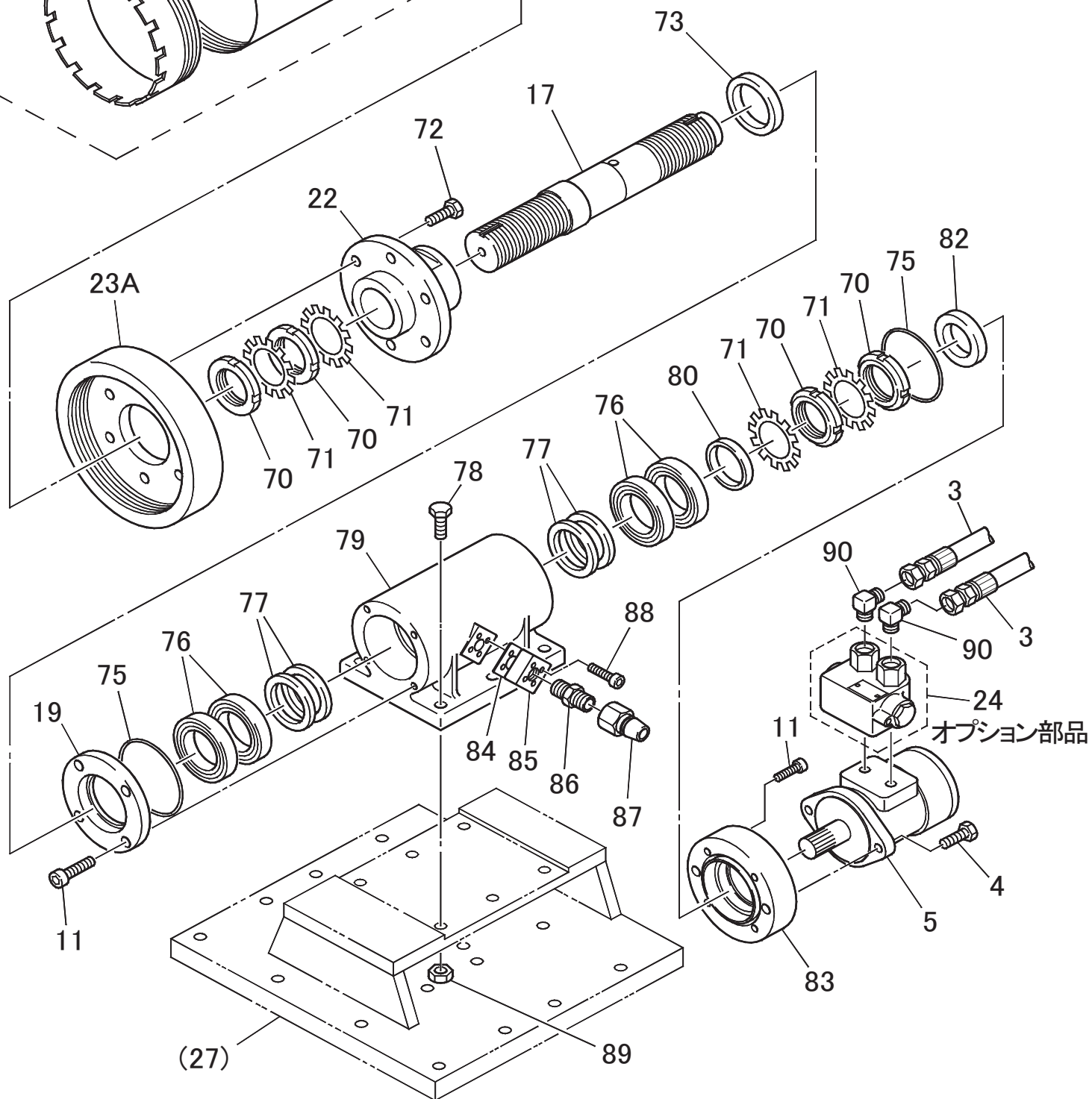
油圧穿孔機～コーアマン～『RDシリーズ』分解図(1/3)
