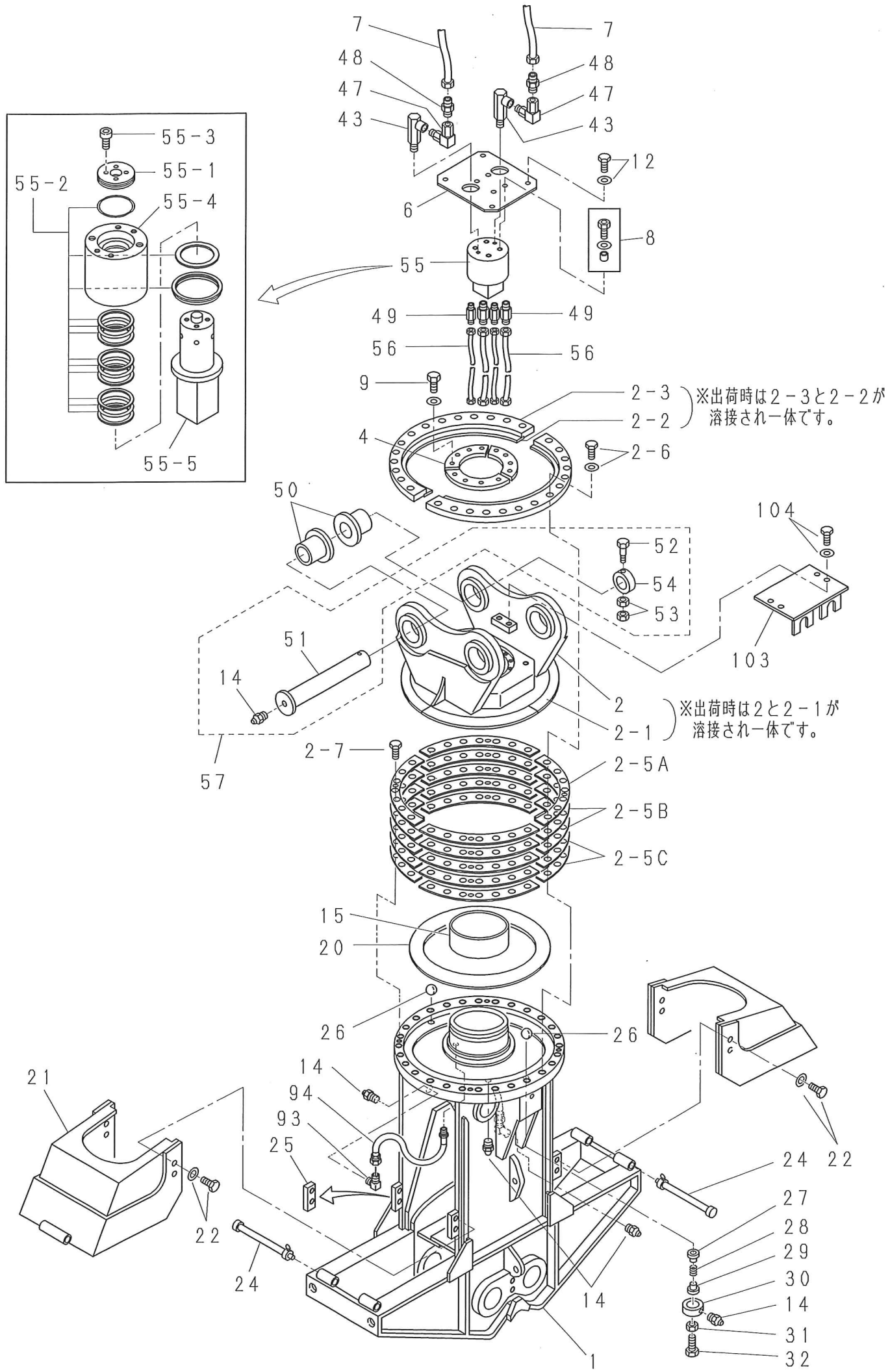
Xカッター 『FE シリーズ』分解図(1/2)
