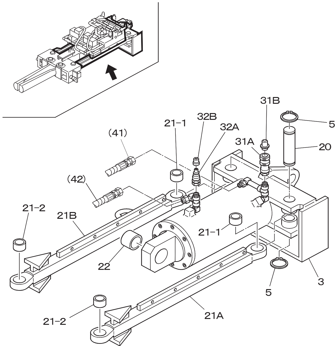
油圧割開機～リキヤ～『HUシリーズ』分解図(2/3)
