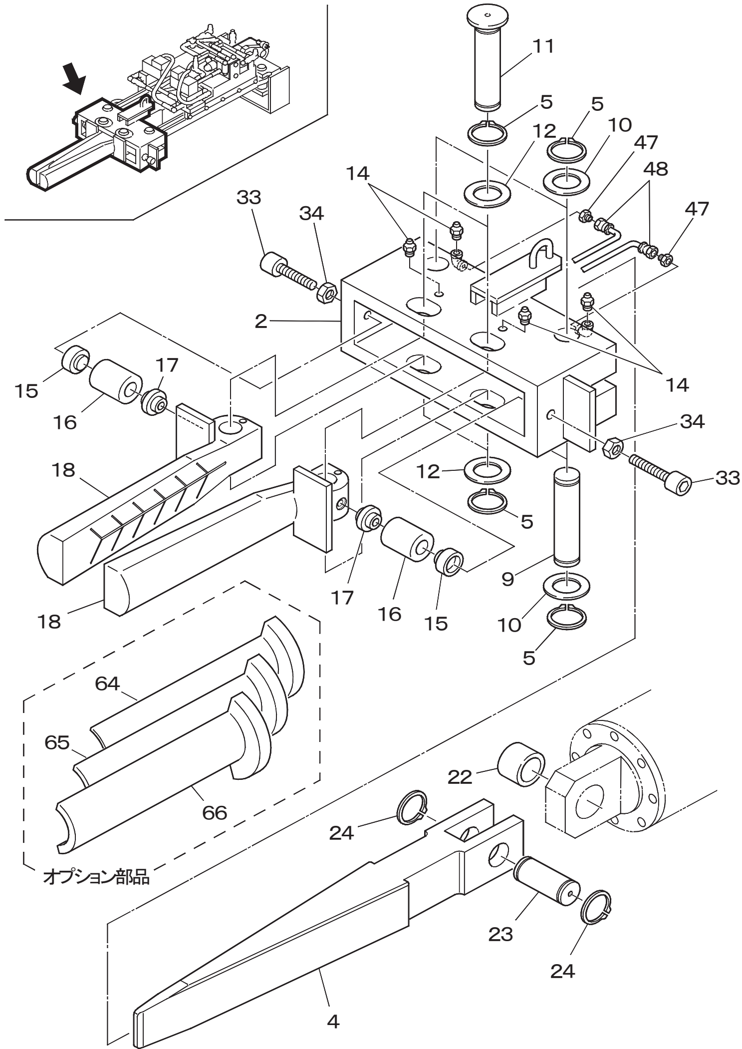
油圧割開機～リキヤ～『HUシリーズ』分解図(1/3)
