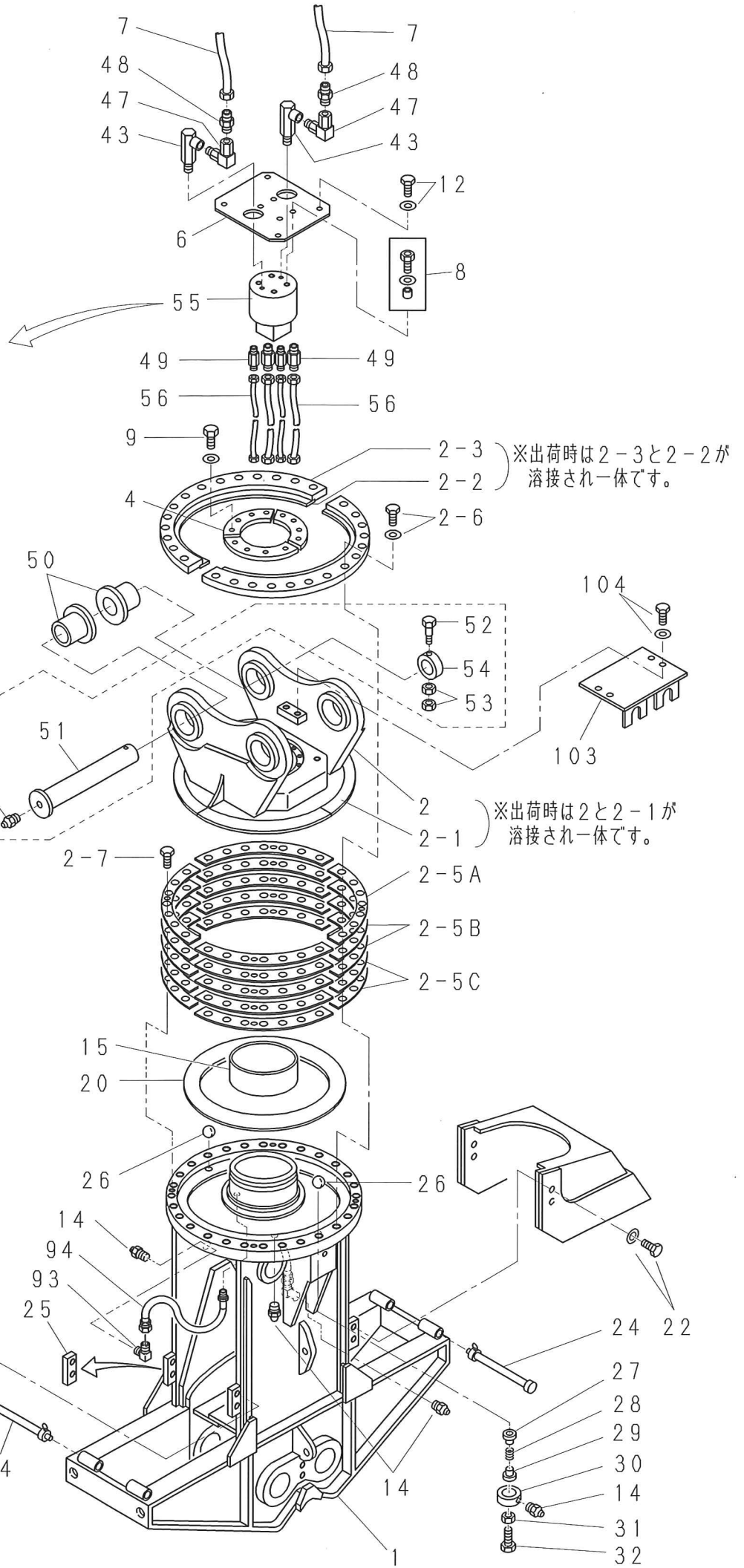
ナンデモカッター『MPCシリーズ』分解図(1/2)
