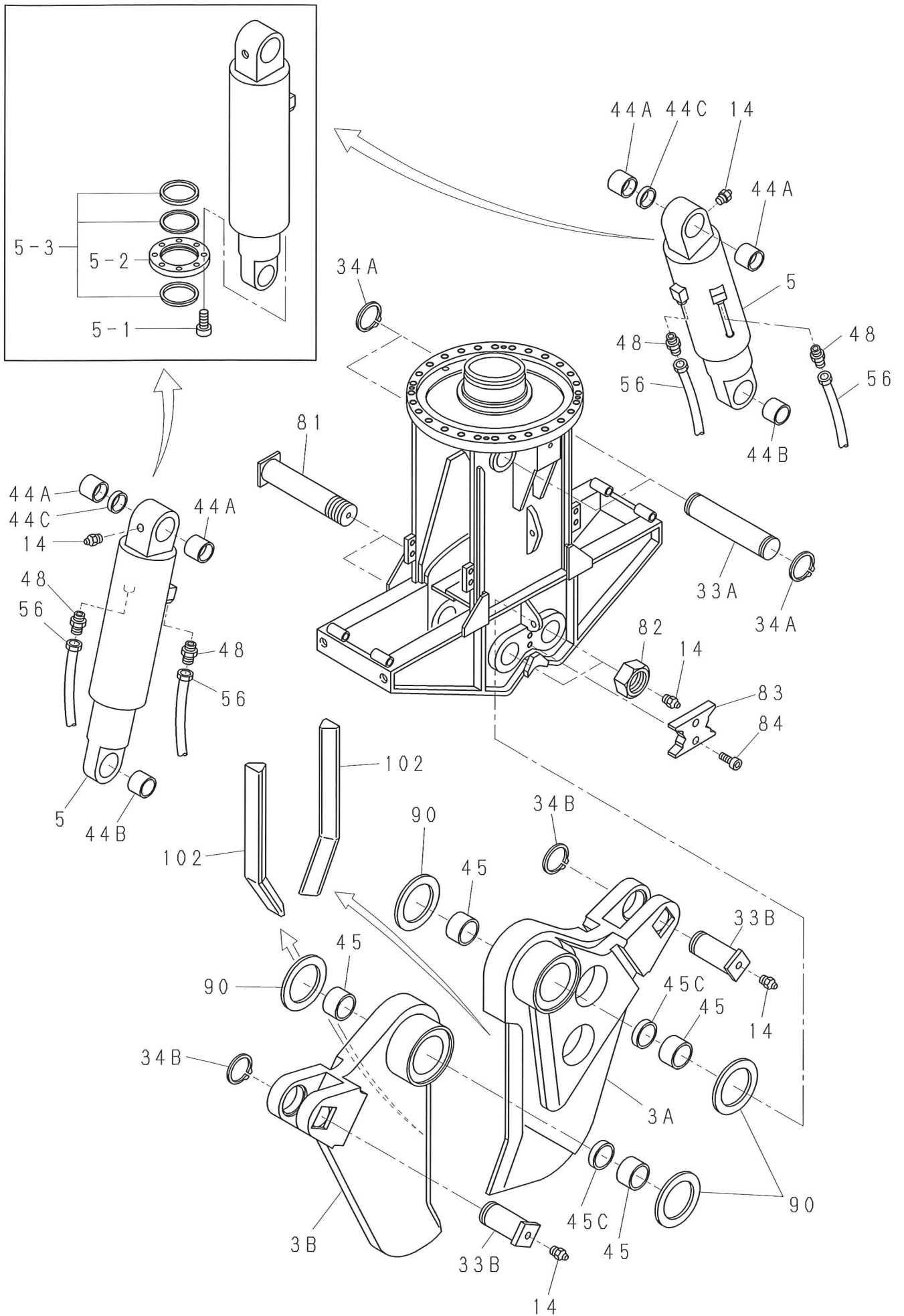
Xカッター 『FE シリーズ』分解図 (2/2)
